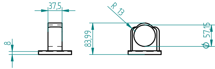
Cilindro buje
