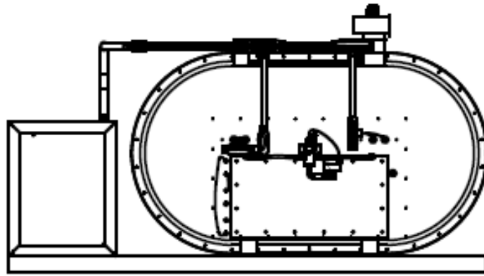
SECTION B-B SCALE 0,09 : 1
