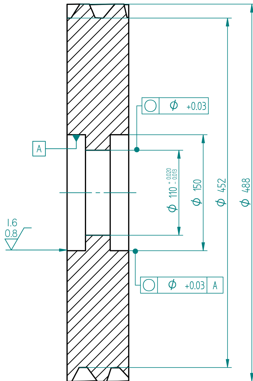
SECTION A-A
