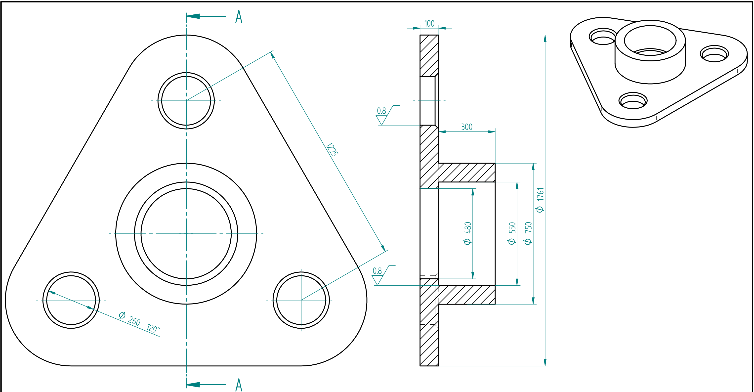
SECTION A-A
