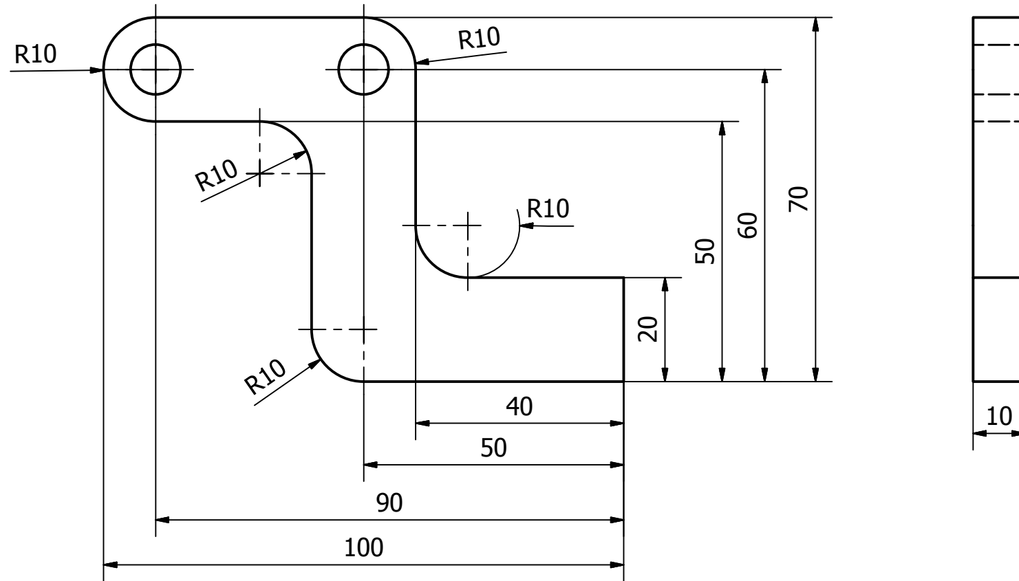
Platina Soporte Caucho Ajuste (E 1:2)
