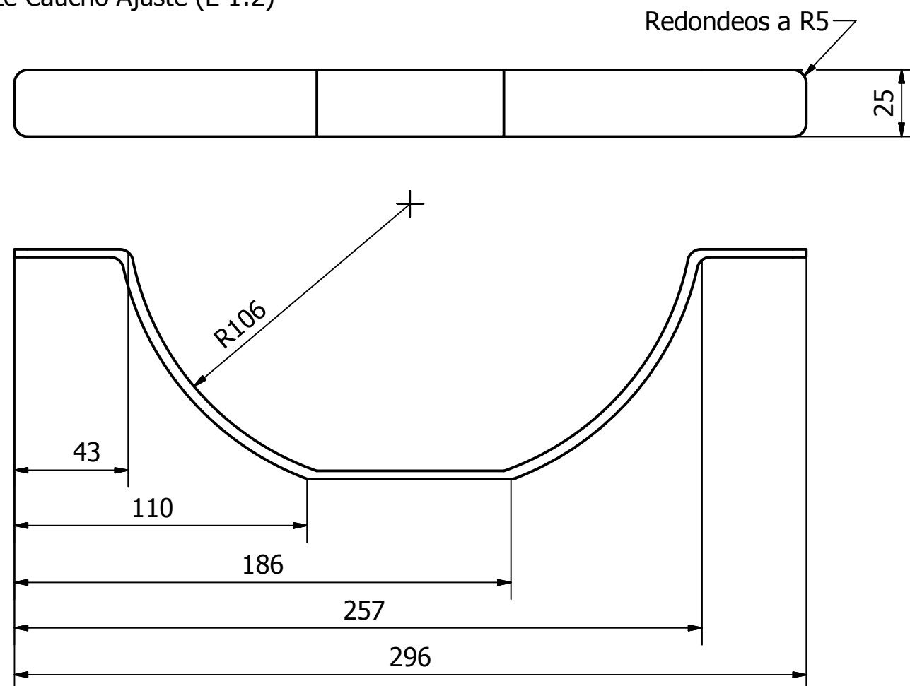
Platina Soporte Caucho Ajuste (E 1:2)
