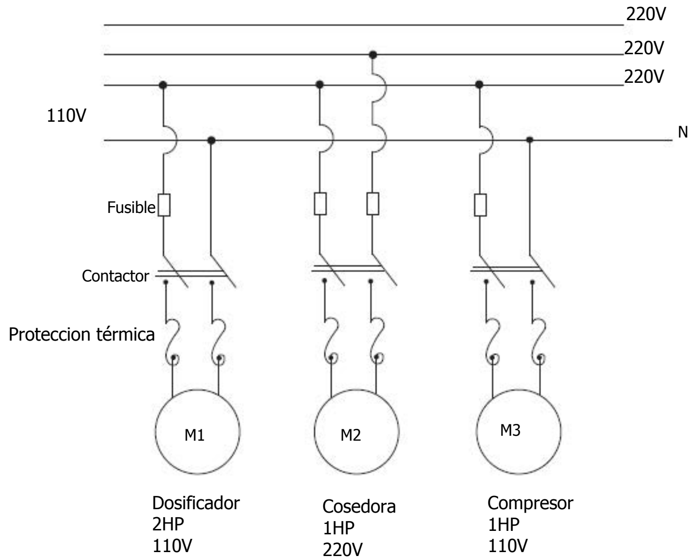
DIAGRAMA DE FUERZA
