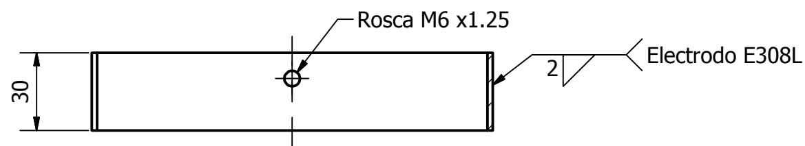
SECTION A-A SCALE 1 : 2
