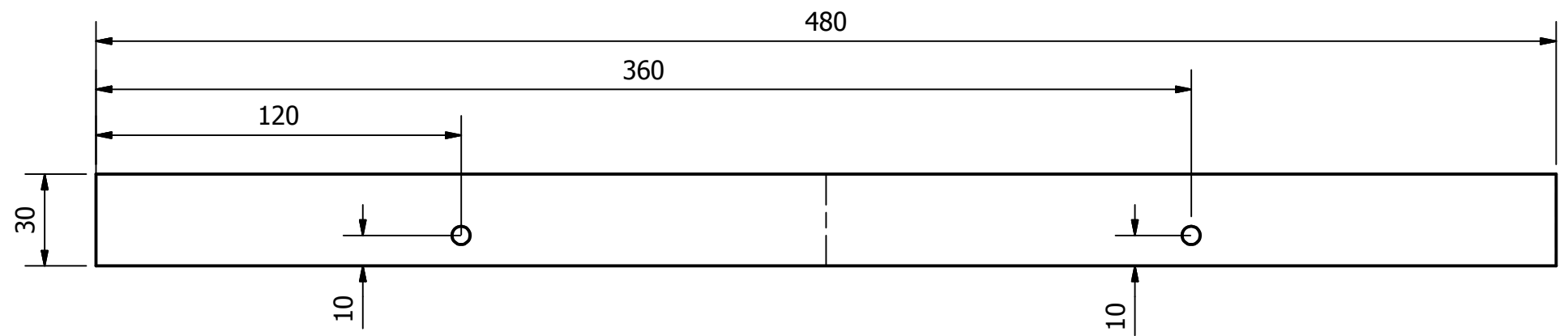
Desarrollo lámina
