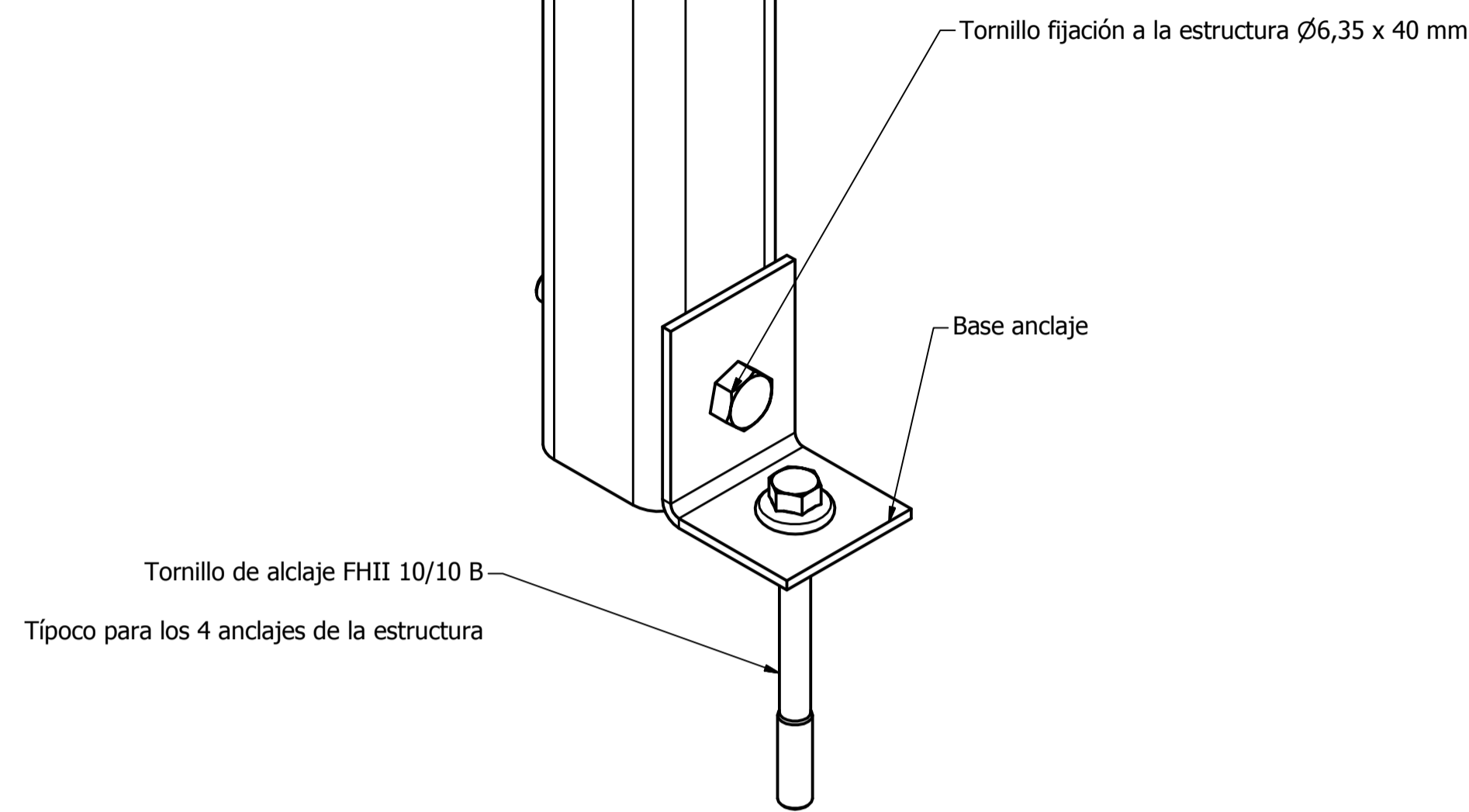
Detalle anclaje al suelo
