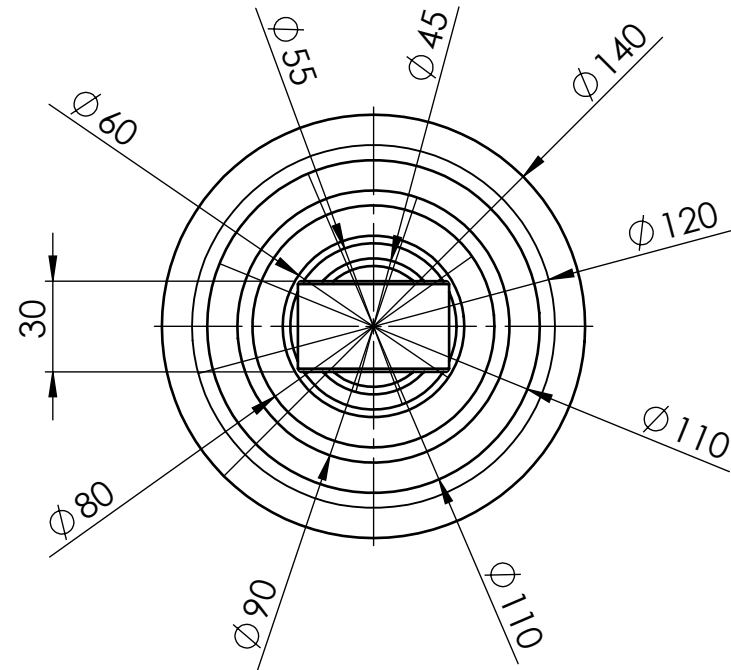
DETALLE A ESCALA 2 : 5
