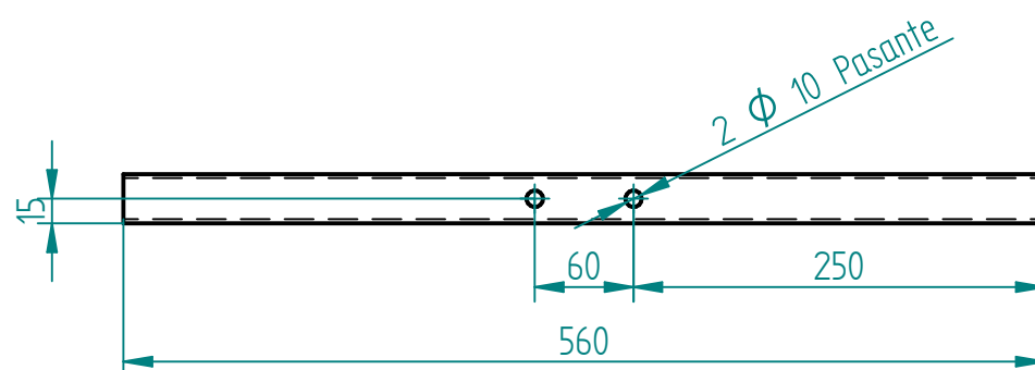
Viga Trasera Motor Escala 1 : 5 Tubo c 30x30x2.5m Acero ASTM A500
