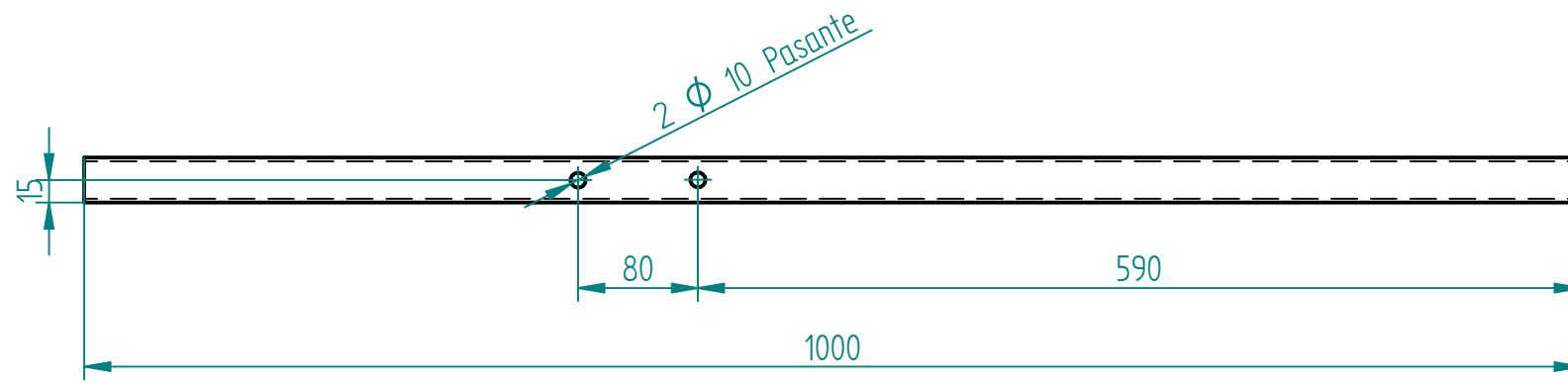
Viga Delantera Motor Escala 1 : 5 Tubo c 30x30x2.5mm Acero ASTM A500
