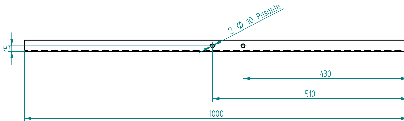
Viga Trasera Motor Escala 1 : 5 Tubo c 30x30x2.5m Acero ASTM A500
