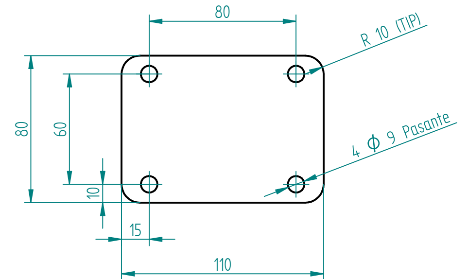
Soporte Ruedas Escala 1 : 2 Acero Galvanizado Lámina rolada en caliente Calibre 13
