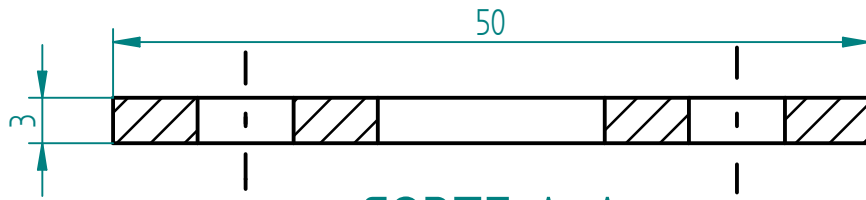
CORTE A-A
