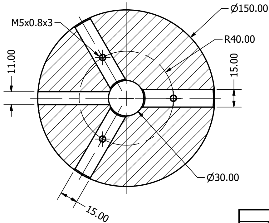
SECCIÓN A-A ESCALA 1 : 2
