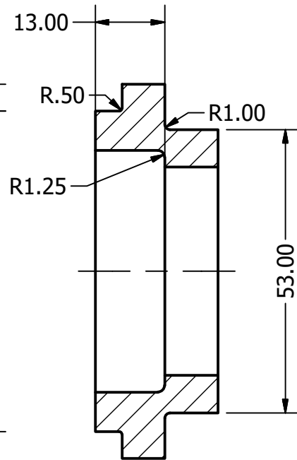
SECCIÓN A-A ESCALA 1 : 1
