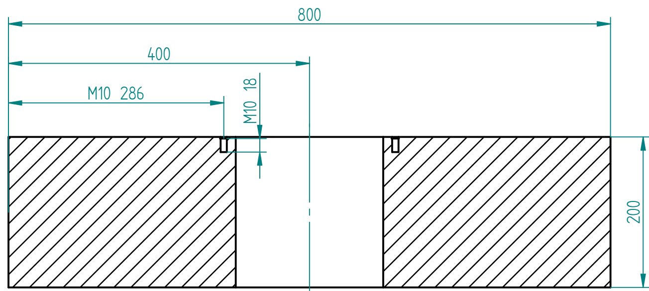
CORTE A-A
