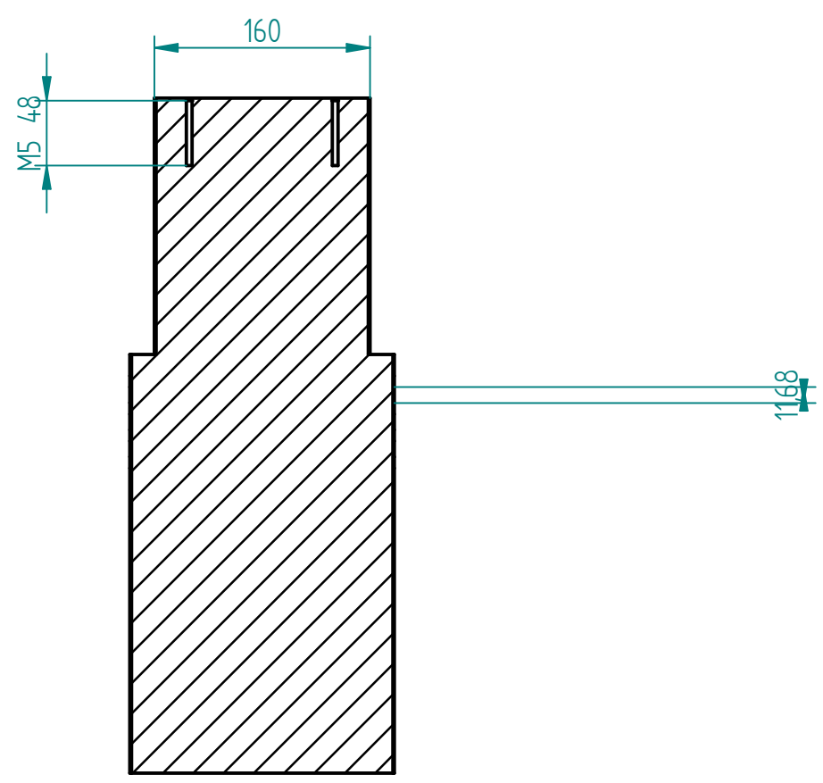
CORTE A-A
