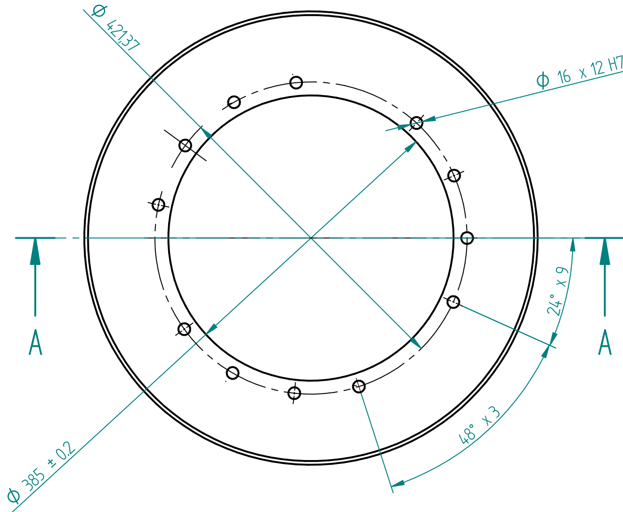
CORTE A-A
