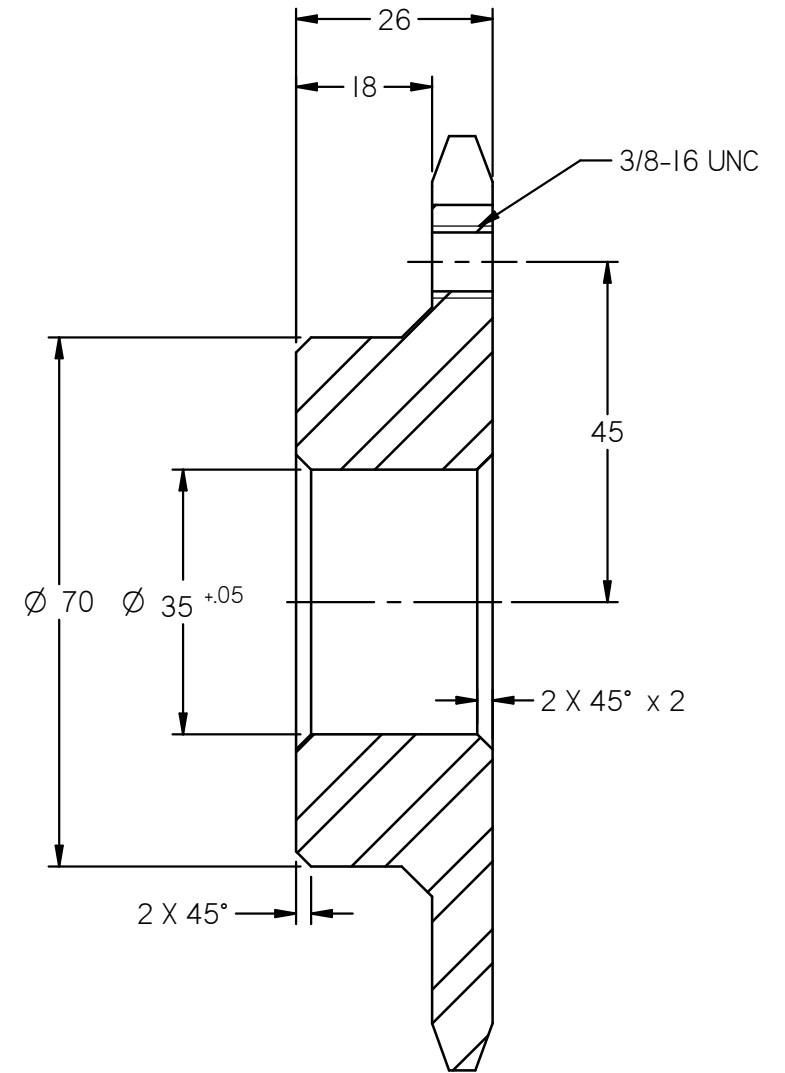
CORTE AH-AH
