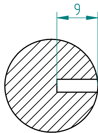
CORTE B-B Escala: 2:1
