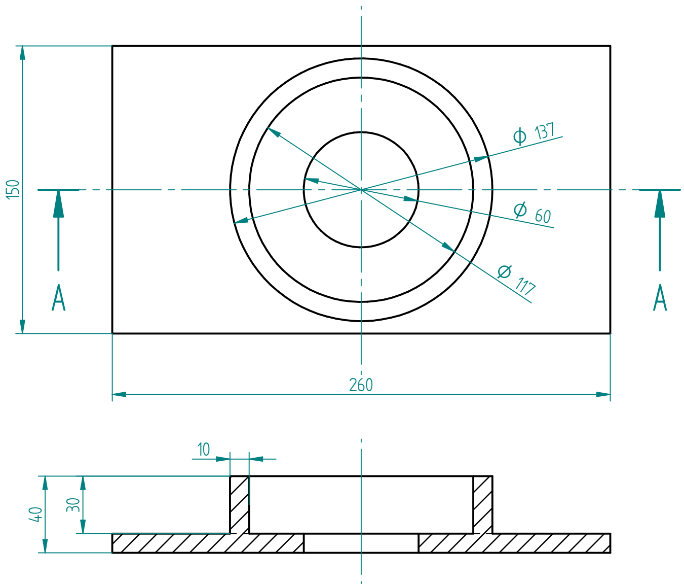
CORTE A-A
