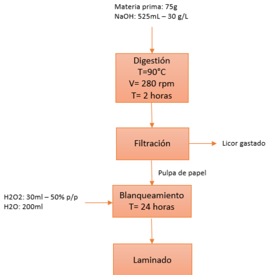
Figura 27. Balance de materia para la obtención de pulpa de papel.
