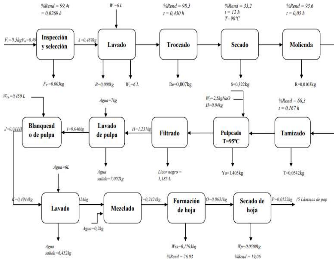
Figura 28. Balance de masas.
