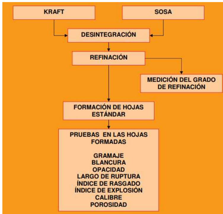
Figura 10. Evaluación físico-mecánica y óptica de la pulpa kraft y a la sosa.
