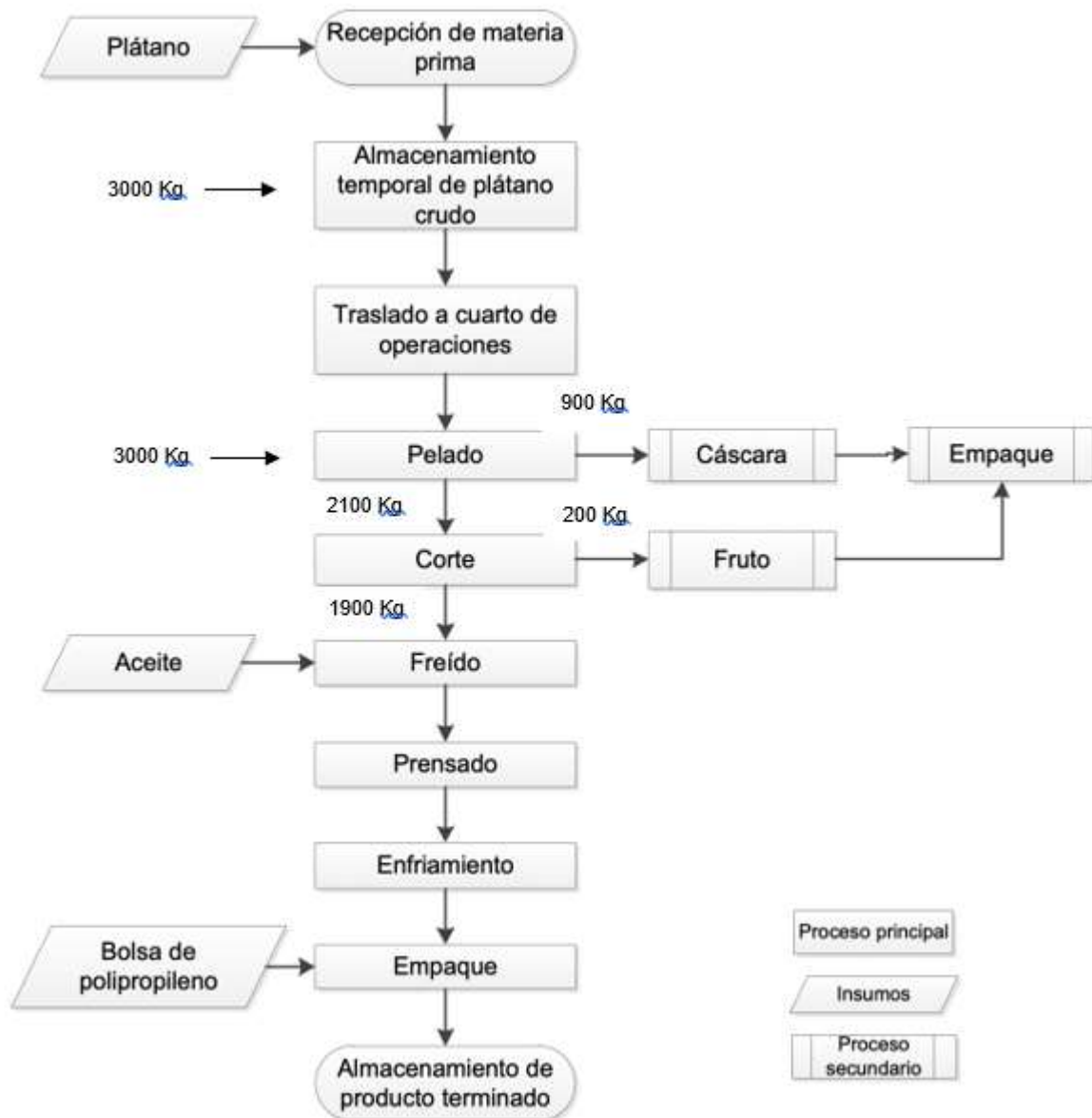
Figura 1. Diagrama de flujo del proceso de producción de la empresa Productos Colombianos S.A.S.
