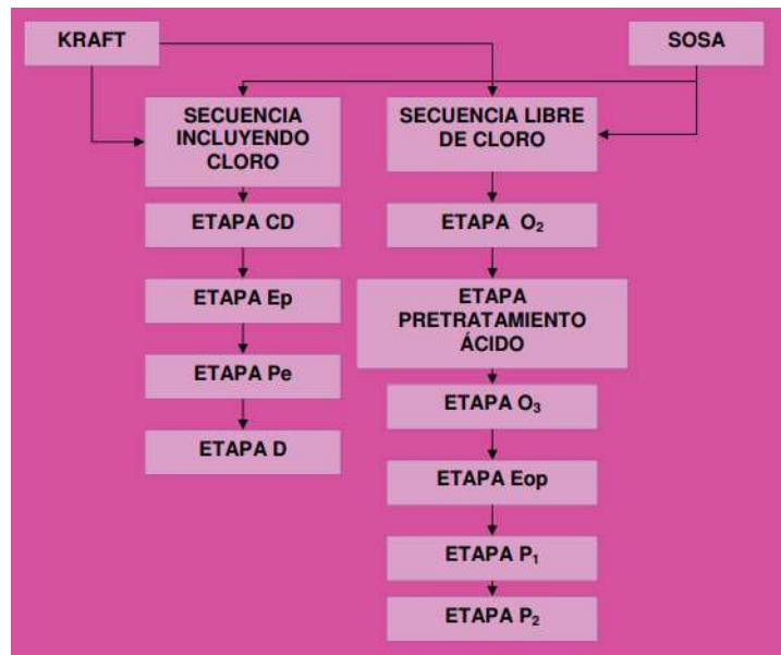
Figura 11. Blanqueo de la pulpa kraft y a la sosa.
