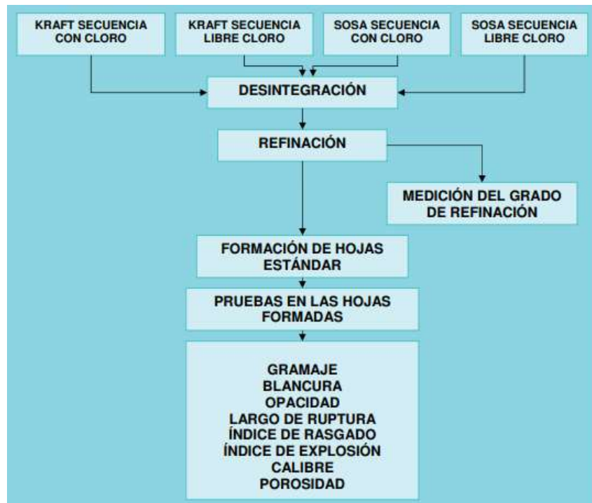
Figura 22. Evaluación fisicoquímica de las pulpas blanqueadas
