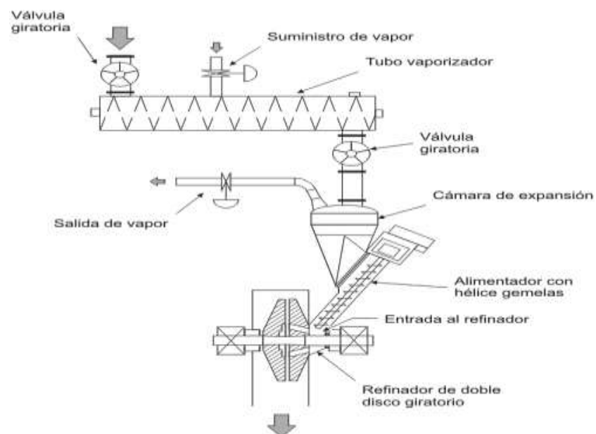
Figura 4. Sistema producción termomecánica de pulpa.
