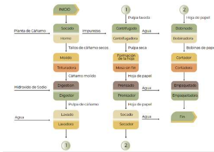
Figura 7. Proceso a la sosa
